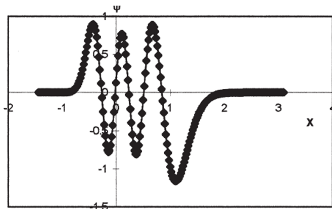
图 13.2: 通过 Numerov 方法求出的 H_2 v = 5 莫尔斯振动波函数。
